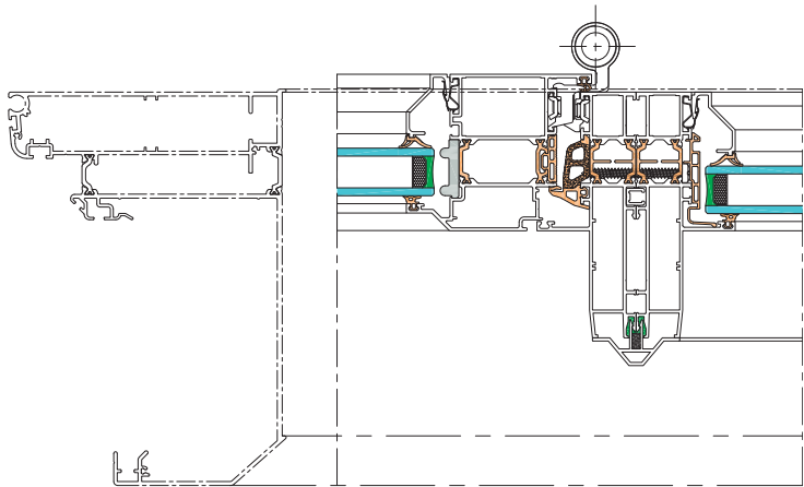
Coupe dormants dos à dos
