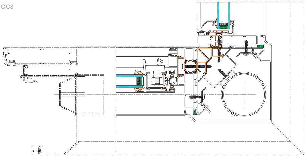
Coupe poteau à 90°
