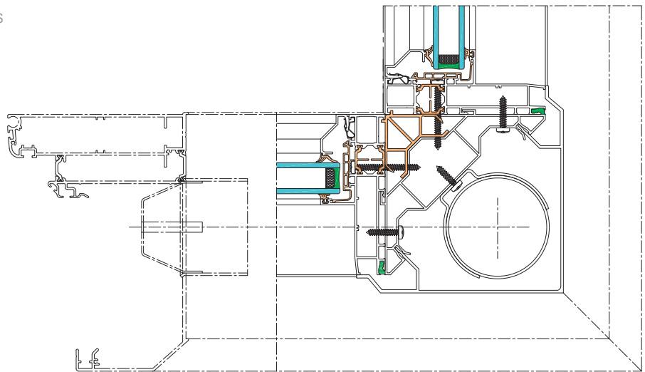
Coupe poteau 90°
