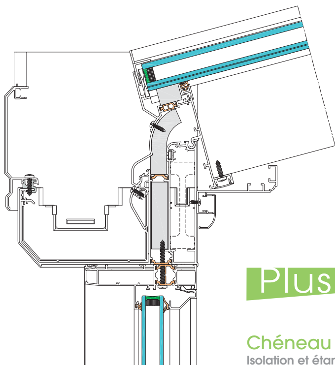
Coupe chéneau
