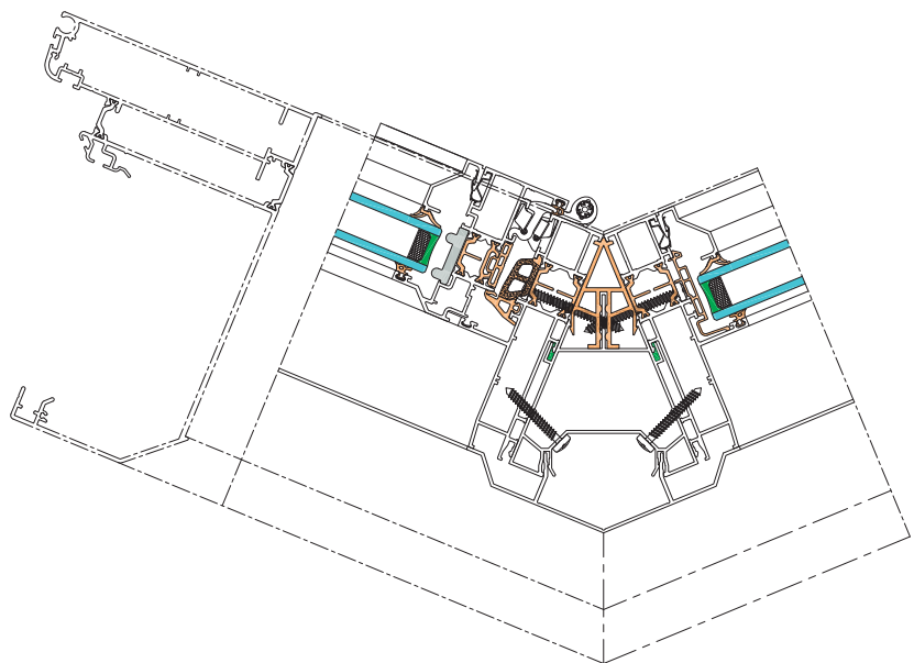
Coupe poteau à 135° ou 150°
