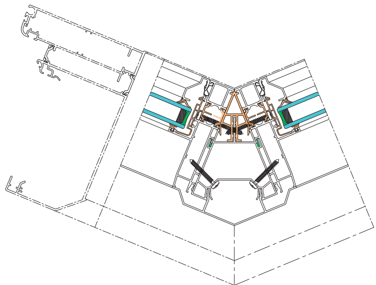
Coupe poteau 135° ou 150°
