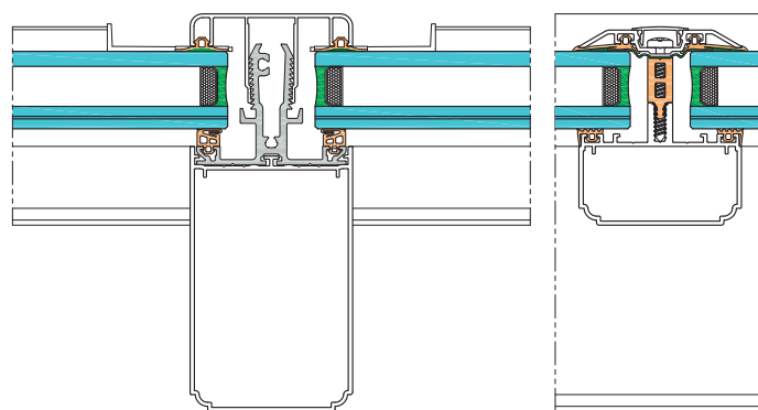
Coupes chevrons
