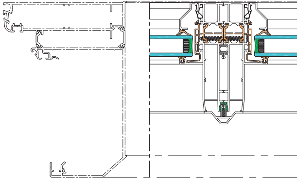
Coupe dormants dos à dos
