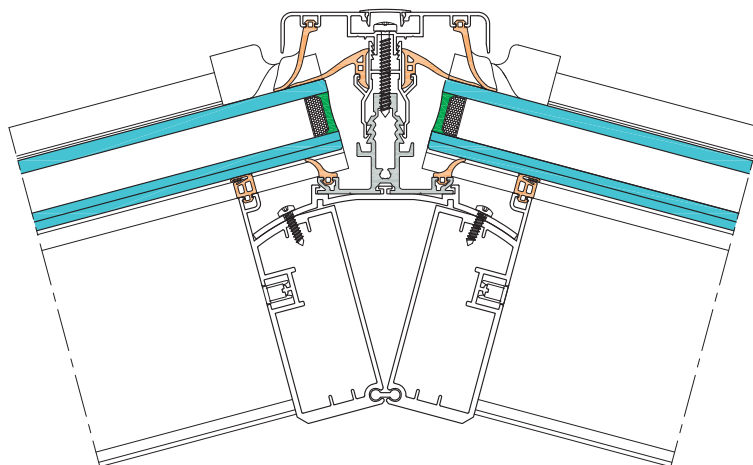
Coupe arêtier
