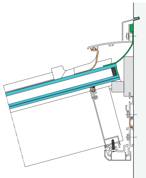
Coupe faîtière
